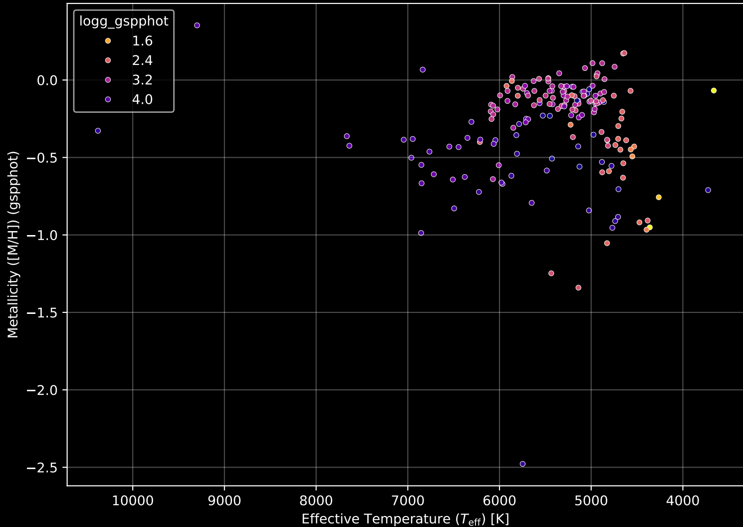
APOGEE DR17 Field: [000+45] Stellar Population Parameters (n= 177)
